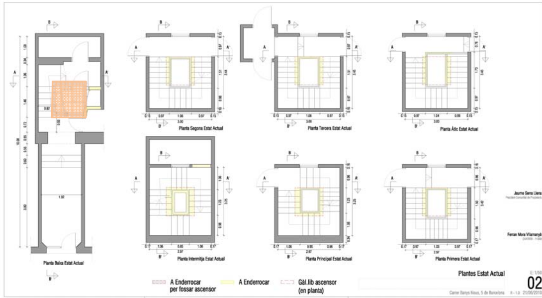
Planta de la finca i situació de la cala.
