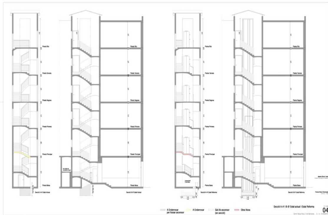
Seccions
